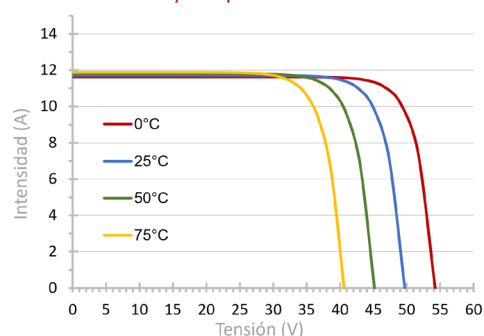
Curvas I-V y Temperaturas °C
